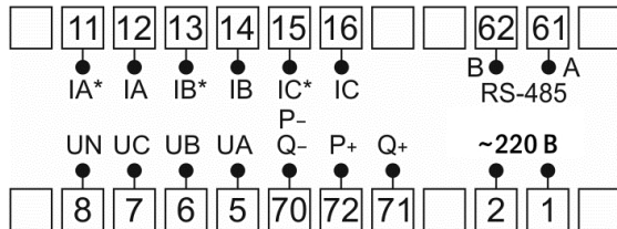
Рис. 3 – Схема подключения
