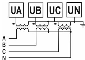
Рис. 5 – Подключение трансформатора напряжения x/380 В (трехфазная цепь с нейтралью)
